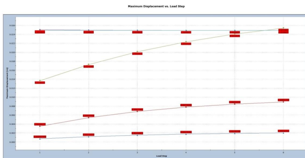
Рисунок 4.37. Смещение (бетон толщиной 35 см) САСТ-5 в разрезе 4
