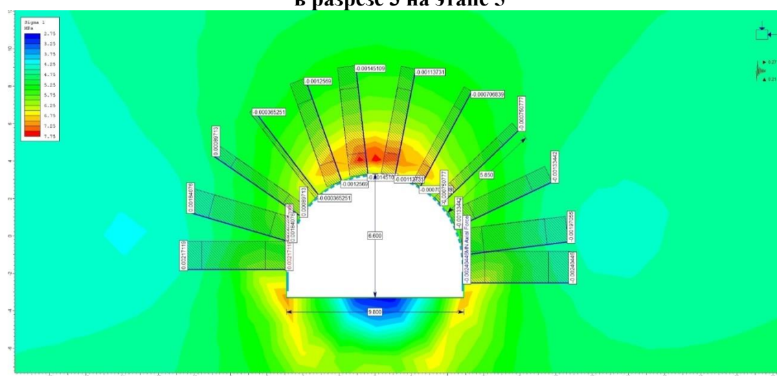
Рисунок 4.27. Осовая сила анкера (торкретбетон, проволоочная сетка и анкера) САСТ-5 в разрезе 3 на этапе 5
