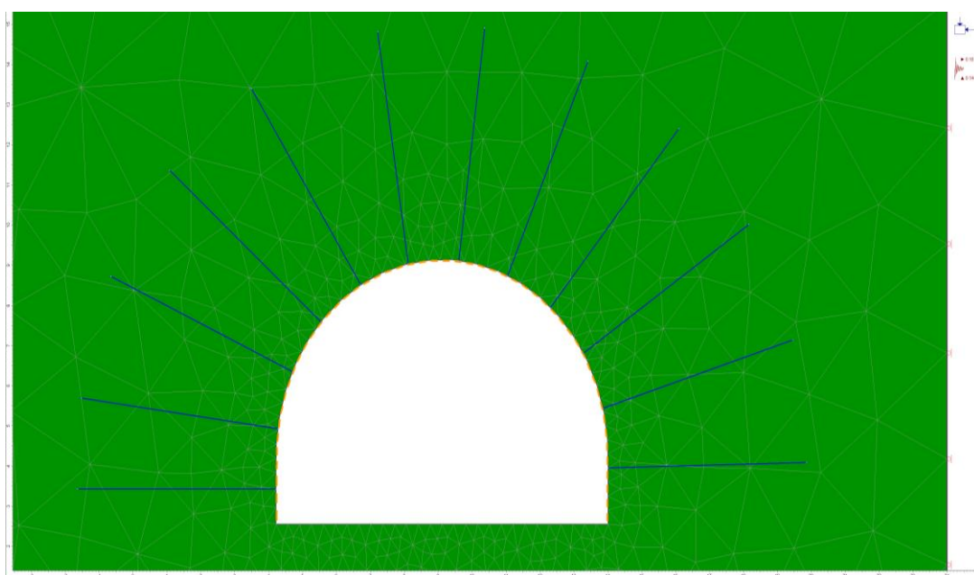
Рисунок 4.22. Крупный вид конечно-элементной модели САСТ-5 в разрезе I (ПК01+84,06) на этапе 5
