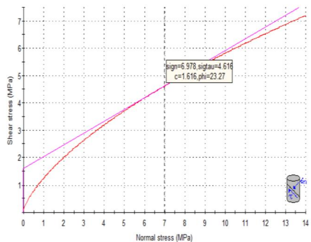
Рисунок 4.2. Механические параметры массива горных пород, окружающего разрез 1.
