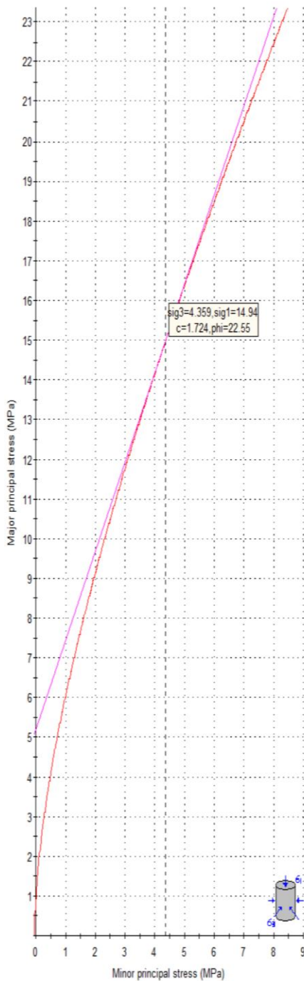
Рисунок 4.2. Механические параметры массива горных пород, окружающего разрез 1.
