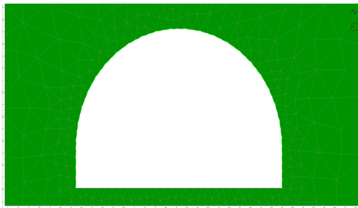
Рисунок 4.13. ТИП-Шб Общий вид КЭ модели САСТ-5 в разрезе 2 (ПК01+100 ~ ПК02+060) на этапе 5
