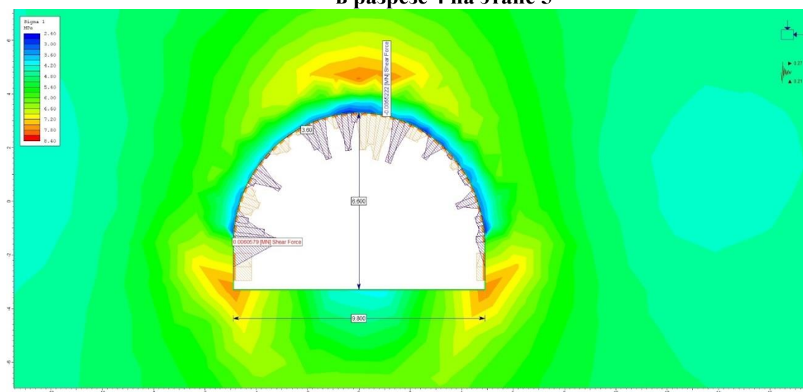
Рисунок 4.36. Сдвигающая сила разрез II – Этап 5 –Элементы текучести вокруг тоннеля
