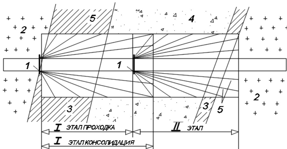
Рисунки 3.2. Схема консолидации раздробленных пород при проходке туннеля ГЭС Розелан-Бати
