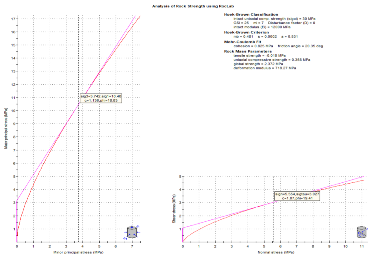
Рисунок 6.47. Показаны механические параметры массива горных пород, окружающего в разрезе 6.
