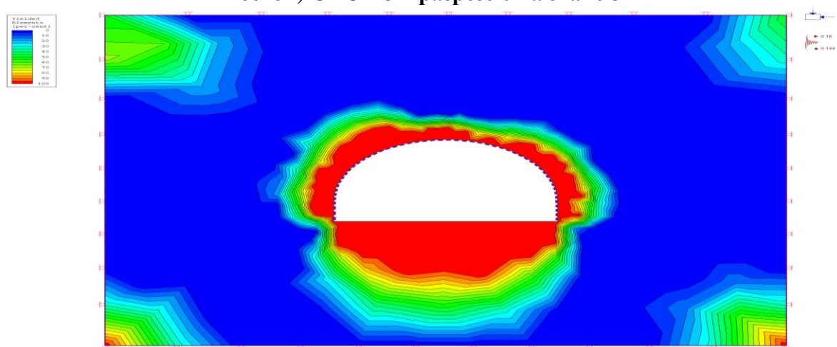
Рисунок 4.54. Элементы текучести обделки (стальные ребра и простой бетон) САСТ-5 в разрезе 6 на этапе 5
