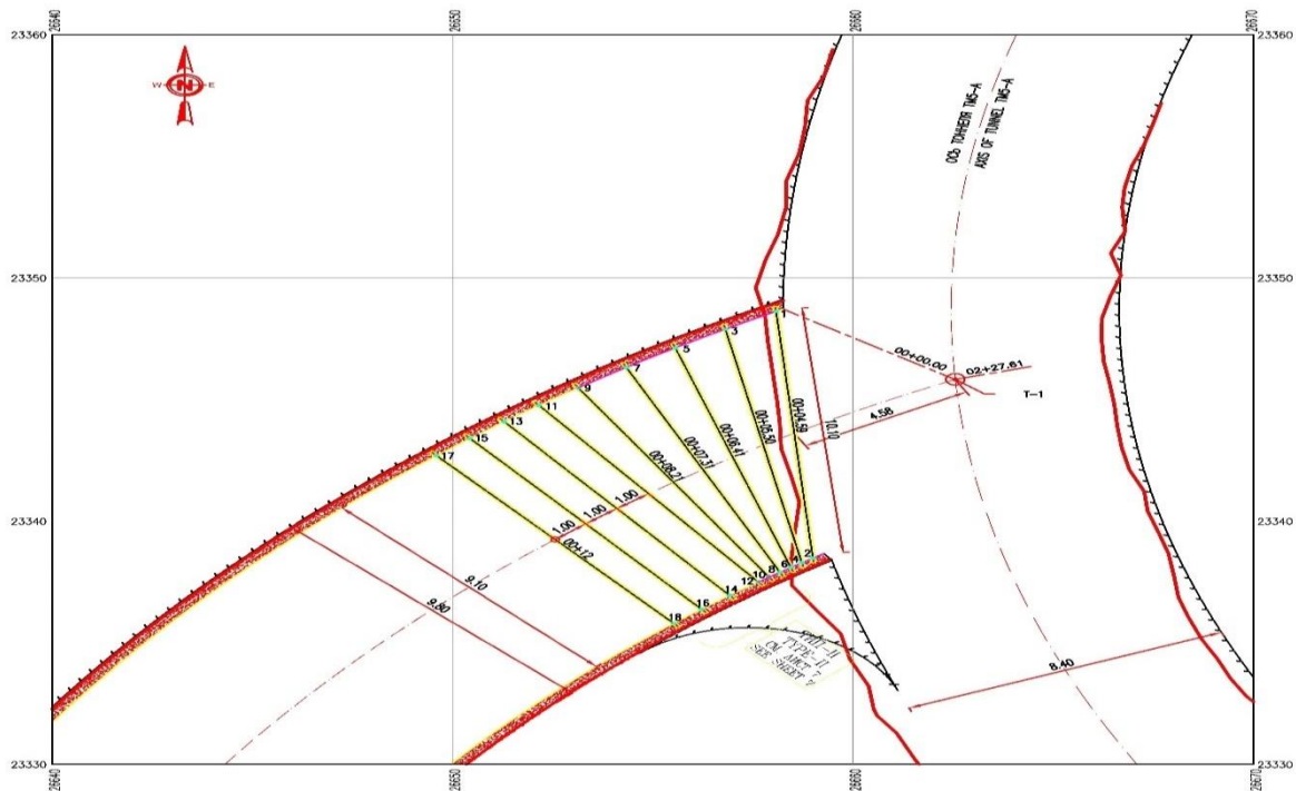
Рисунок 2.5. Соединение тоннеля TM5-A и САСТ-5
