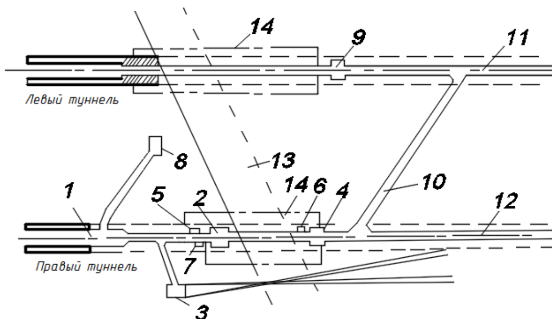
Рисунки 3.3. Схема консолидации и проходки зоны разлома при строительстве Гран-Сасского тоннеля. 1 –ось тоннеля; 2- камера; 3 – дренажная камера; 4 –7- рабочая камера; 8-камера оборудования; 9 – камера; 10 – рассечка; 11 -12 – пилот-тоннеля; 13-зона разлома; 14 –укрепительные породы.
