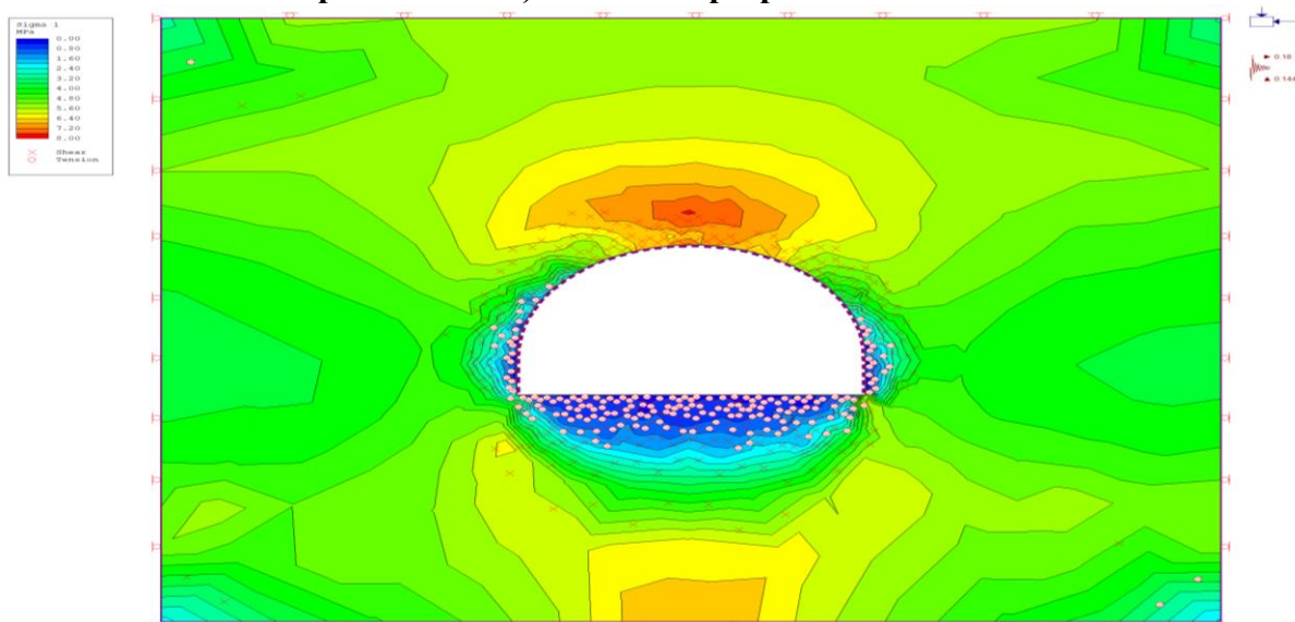
Рисунок 4.51. Sigma 1 и элементы текучести обделки САСТ-5 в разрезе 6 на этапе 5
