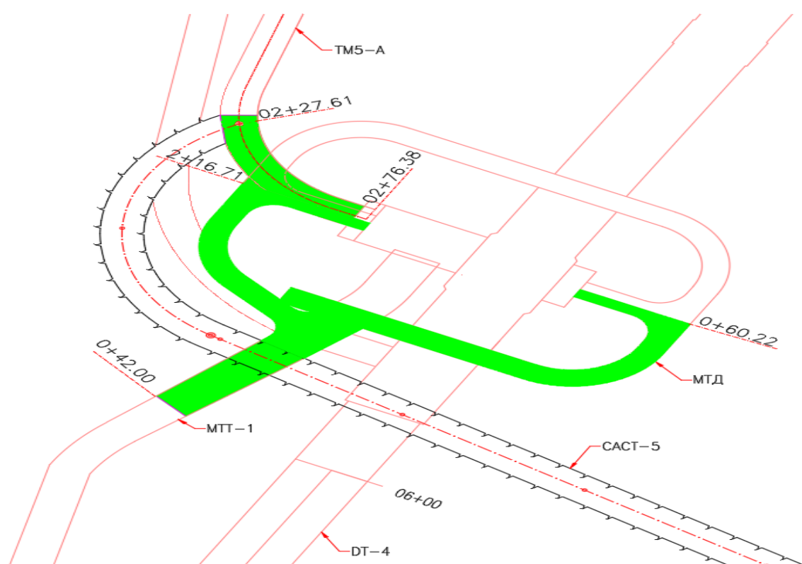
Рисунок 2.9. Расположение участков тоннелей ТМ5-А, МТТ-1 и МТД, инженерно-геологическое картирование которых использовалось для инженерной классификации горных массивов вдоль штольни САС-5.
