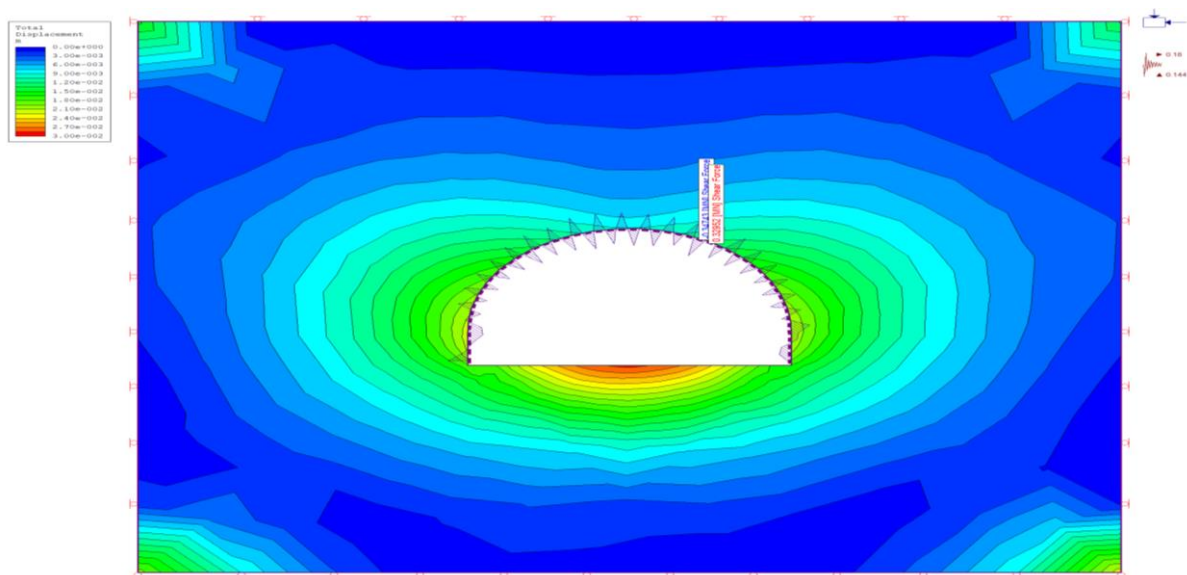
Рисунок 4.62. Общие смещение и сдвига обделки (стальные ребра и простой бетон) САСТ-5 в разрезе 7 на этапе 5
