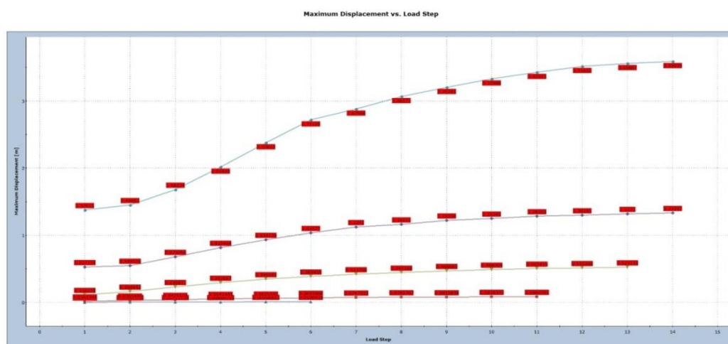
Рисунок 4.45. Смещение (стальные ребра и простой бетон) САСТ-5 в разрезе 5 на этапе 5
