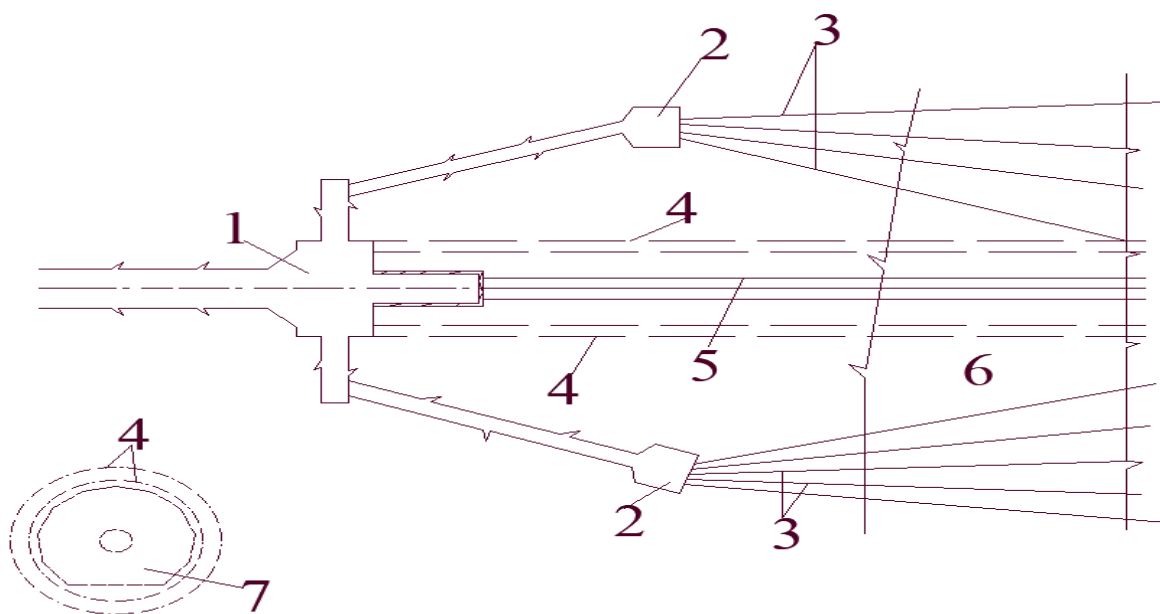
Рисунки 3.8. Консолидация зоны сброса при проходке тоннеля Мантаро.
