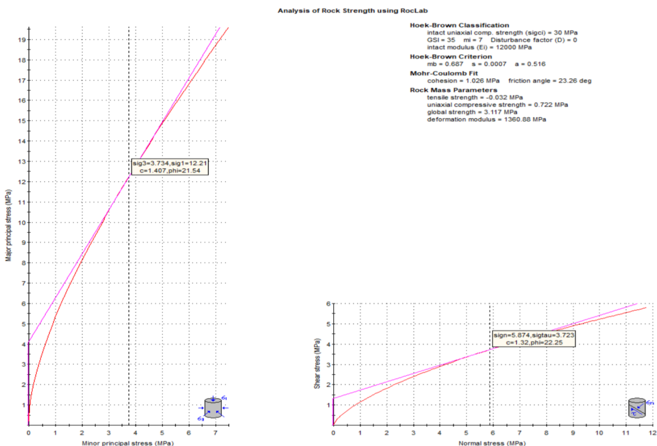
Рисунок 4.56. Механические параметры массива горных пород, окружающего разрез 7
