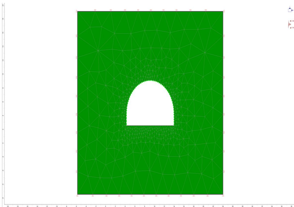
Рисунок 4.12. ТИП-Шб Общий вид КЭ модели САСТ-5 в разрезе 2 (ПК01+100~ПК02+060) на этапе 5
