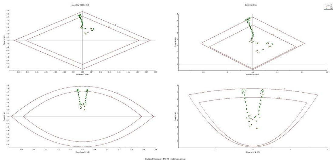
Рисунок 4.46. Несущая способность обделки (стальные ребра IPE 240 мм и обычный бетон 30 см) САСТ-5 в разрезе 5
