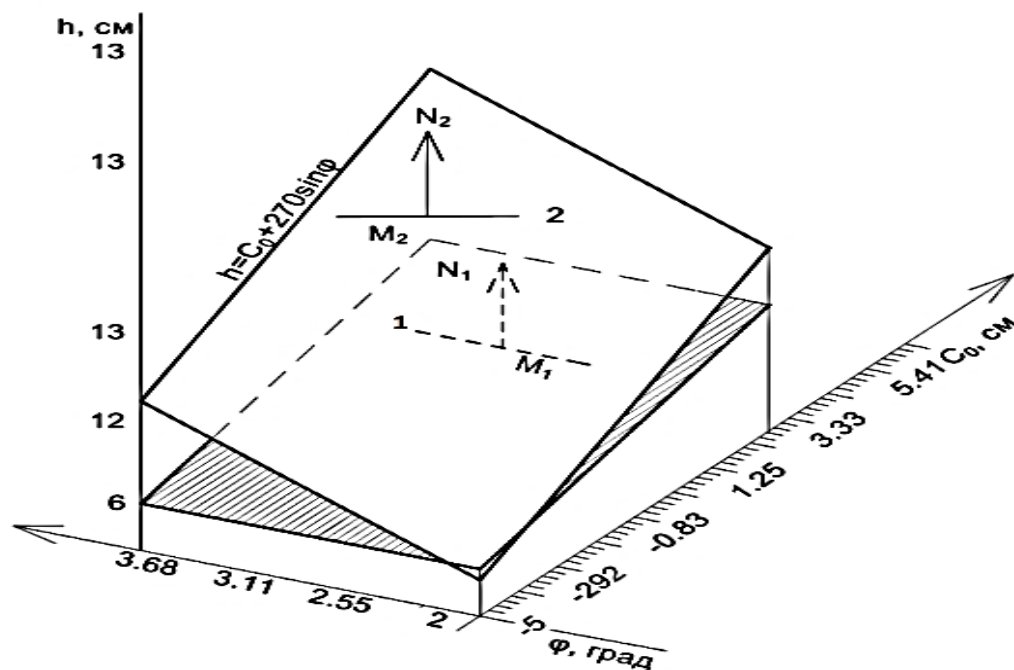
Рисунки 3.6. Графическое сопротивление функциональной (1) и корреляционной (2) зависимости законтурных переборов h от величины отклонения устья шпуров C_0 и угла наклона их \varphi к проектной поверхности выработки
