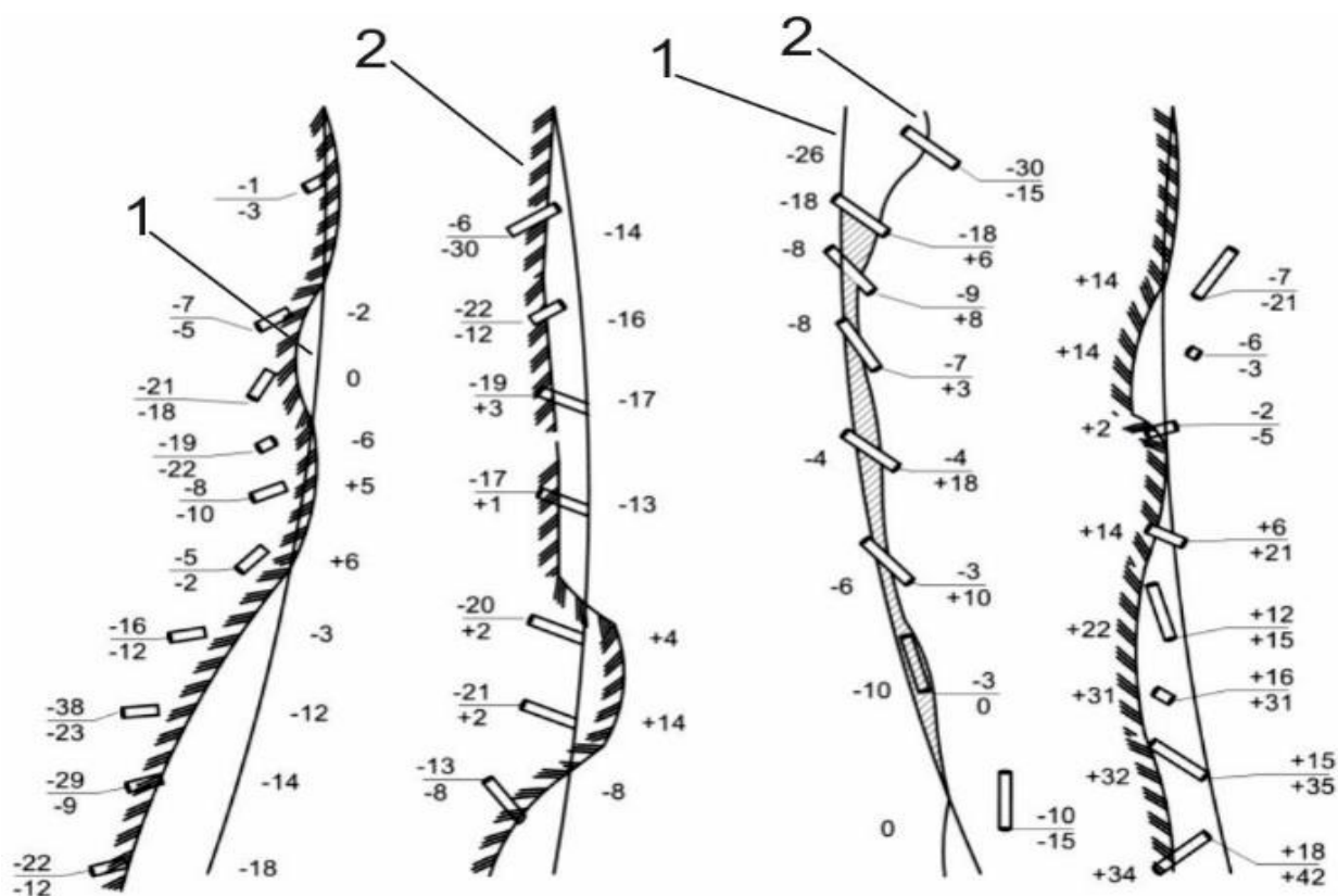
Рисунок 3.4. Результаты забойных измерений параметров контурных шпуров:
