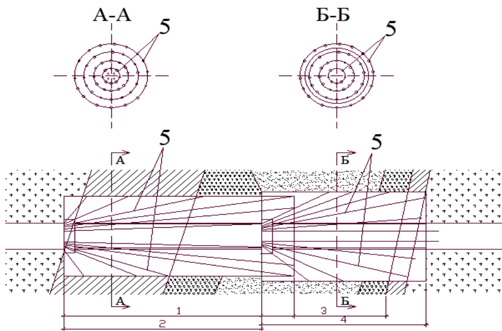
Рисунки 3.7. Схема консолидации раздробленных пород при проходке тоннеля Розелан-Бати
